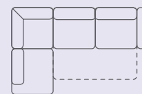
OTL + 2,5 FP Šírka 247 cm, hĺbka 235 cm. Rozmer po rozložení 190 x 112 cm
